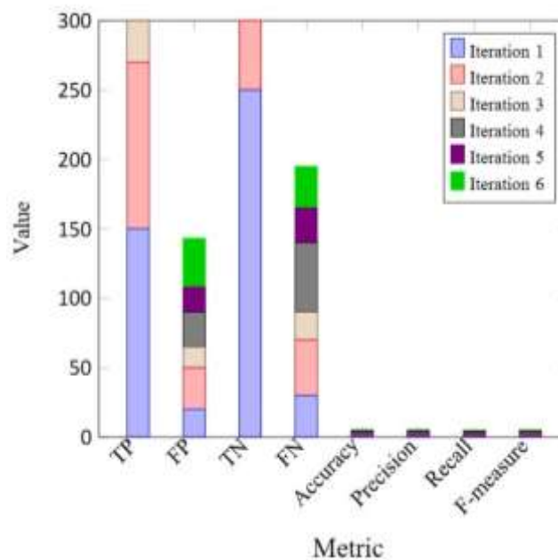
Fig. 3. Precision Metrics
