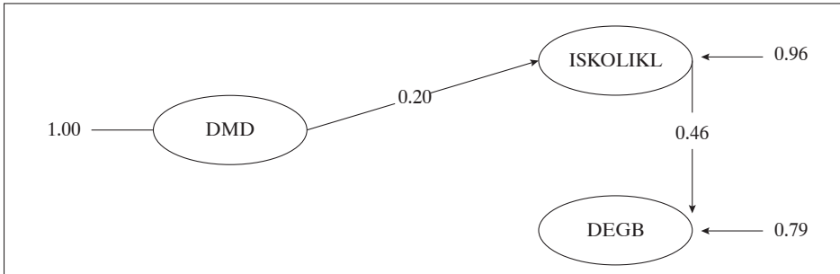
Şekil 12. Model 3'e ait 2. aşama yol analizi
