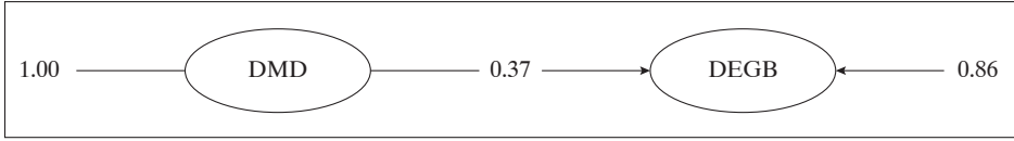
Şekil 11. Model 3'e ait 1. aşama yol analizi
